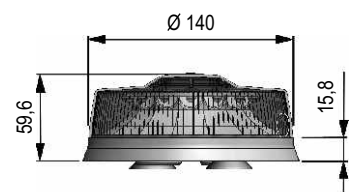
LM400 SOLARIS Abmessungen in mm
