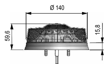
LP400 SOLARIS Abmessungen in mm
